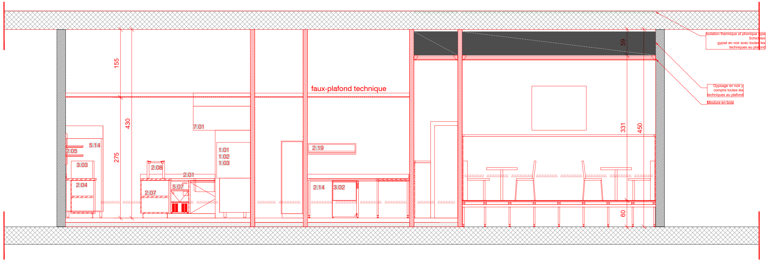
COUPE C
